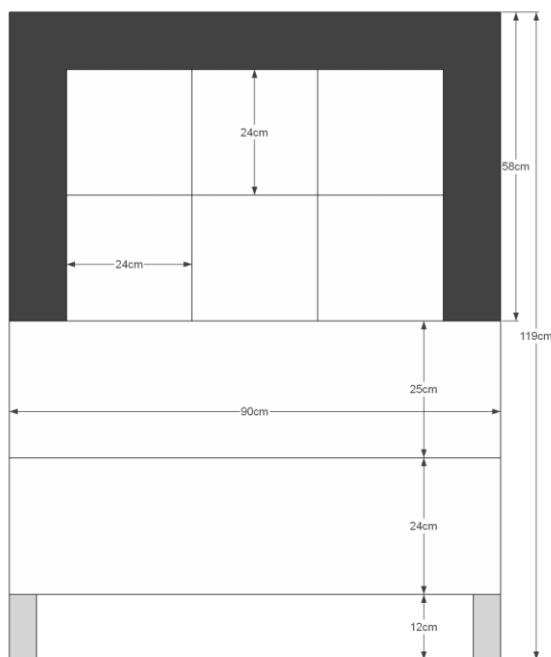
Rysunek nr 1: łóżko wraz z materacem (przekrój pionowy)
