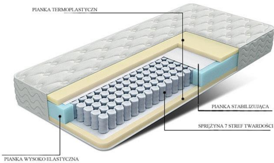
Rysunek nr 3: przekrój materaca
